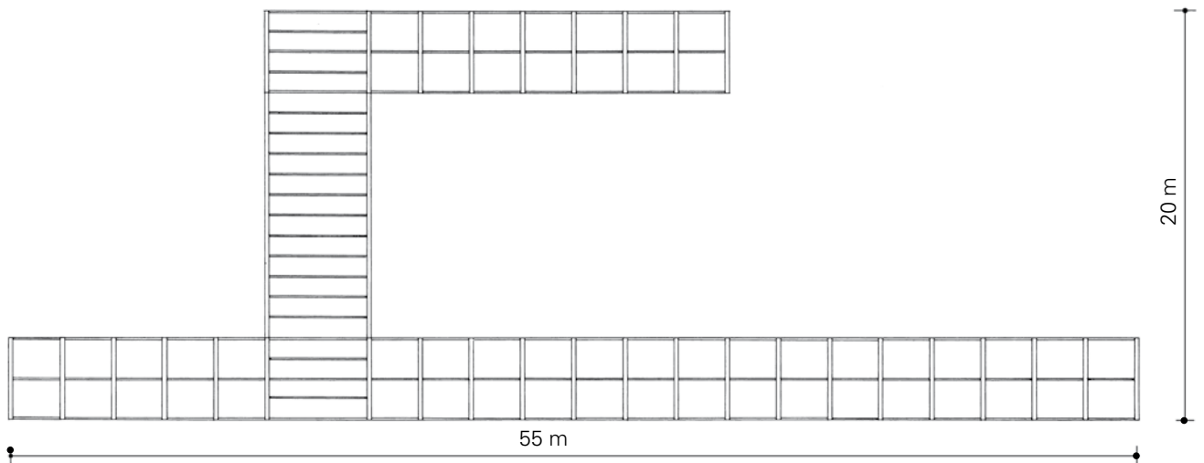
Plattegrond
